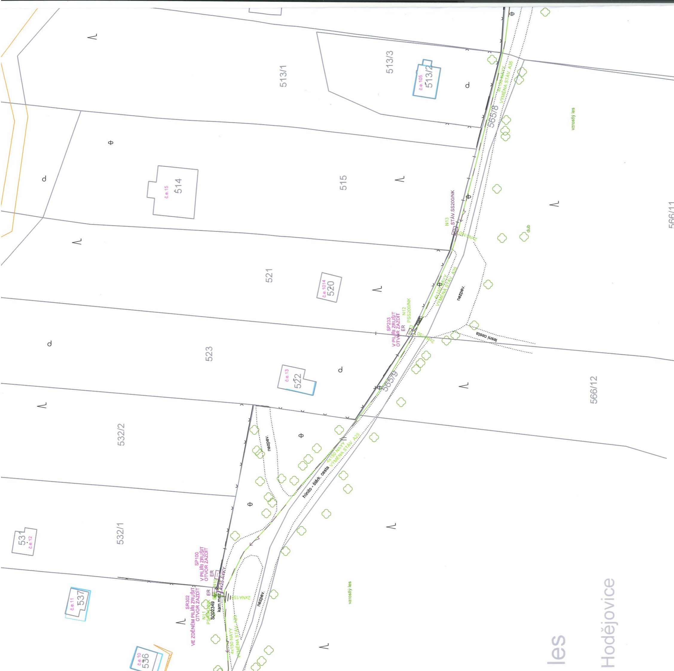
ULOŽENÍ KABELU VN + HDPE CHODNÍK (VOLNÝ TERÉN)
